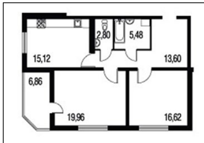
Основной этаж
